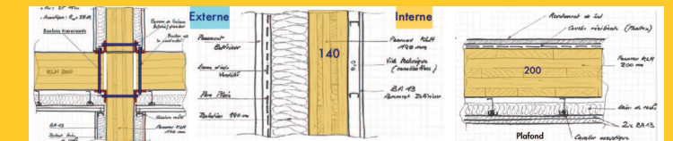
Eléments de construction en bois et assemblages
